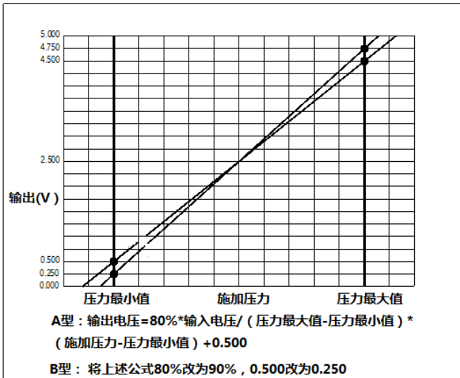
压力转换方程，电压输入5V
