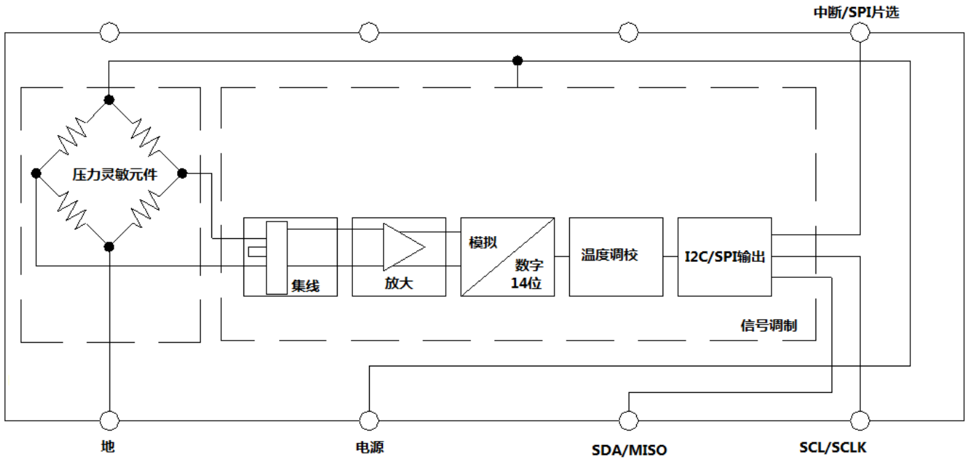
LP55 数字输出等效电路
