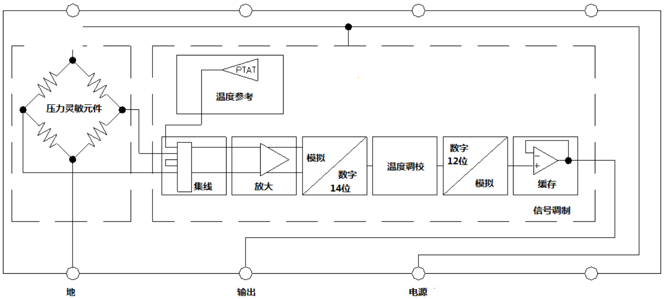
LP55 模拟放大输出等效电路
