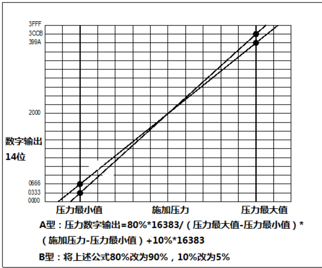
压力转换方程
