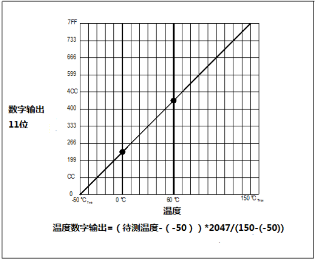
温度转换方程
